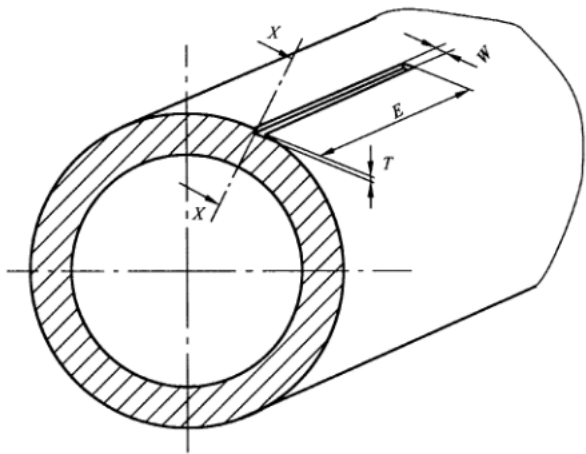
图 C.1 筒体/瓶底过渡区
